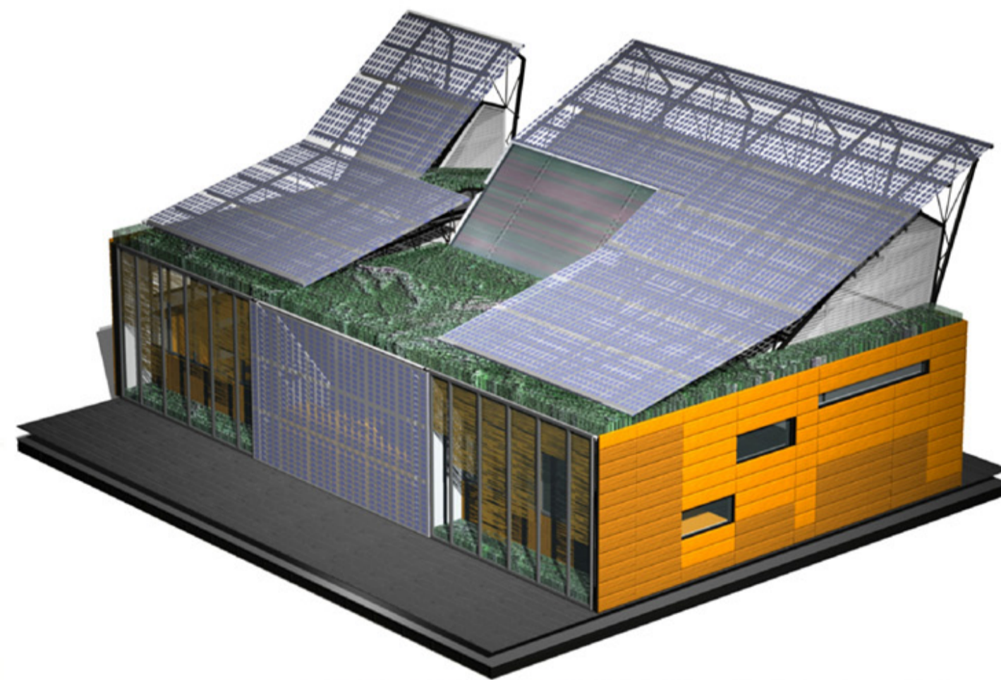
MAGIC BOX: PROYECTO DE CASA SOLAR PRESENTADA POR LA UPM EN EL CONCURSO SOLAR DECATHLON 2005.
